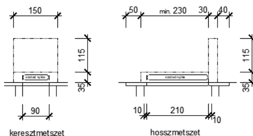
Különálló sírboltra építhető emlék maximális befoglaló méretei
