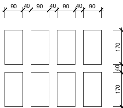
Gyermek sírhelyre építhető járda méretei
