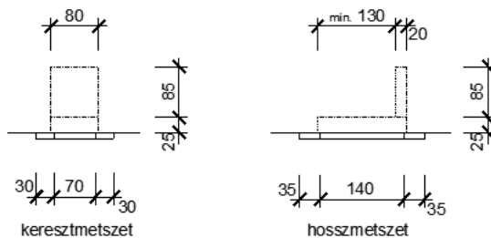
Gyermek sírhelyre építhető emlék maximális befoglaló méretei
