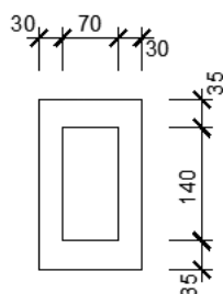
Gyermek sírhelyre építhető emlék maximális befoglaló méretei
